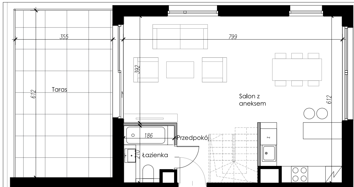
Rzut 4 piętra
